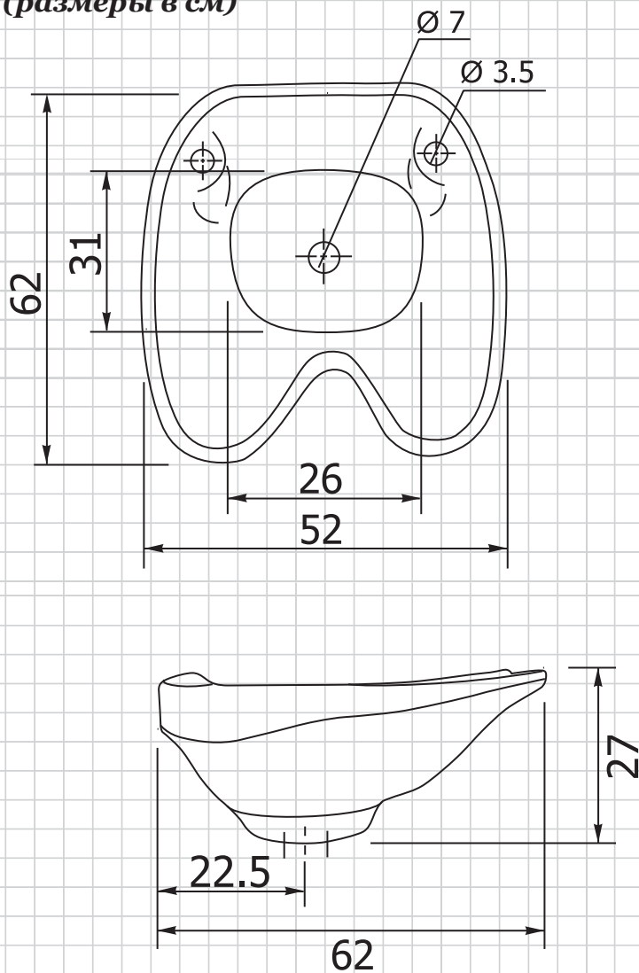
Чертеж раковины (размеры в см)
