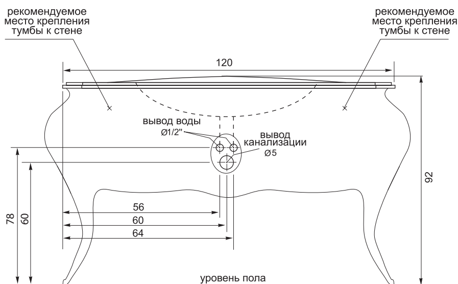
Вывод канализации (рис 1.)
