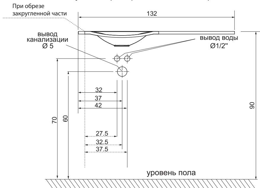
Вывод канализации (рис. 1.)
